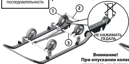
Рис. 3 Механизм выдвигающих колёс
